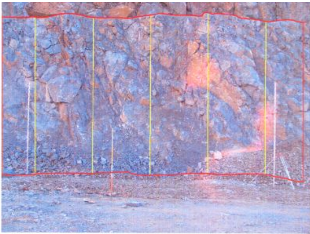
Beispiel für eine Vermessene Wand mit eingezeichneten Bohrlöchern und aufgestellten Meßlatten Gelbe Linien: Beispiele für Bohrlöcher (Sollvorgabe) Rote Linie: Begrenzung der Messfläche (Sprengbereich)
