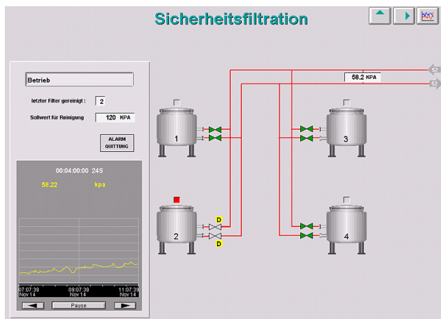
Sicherheitsfiltration
